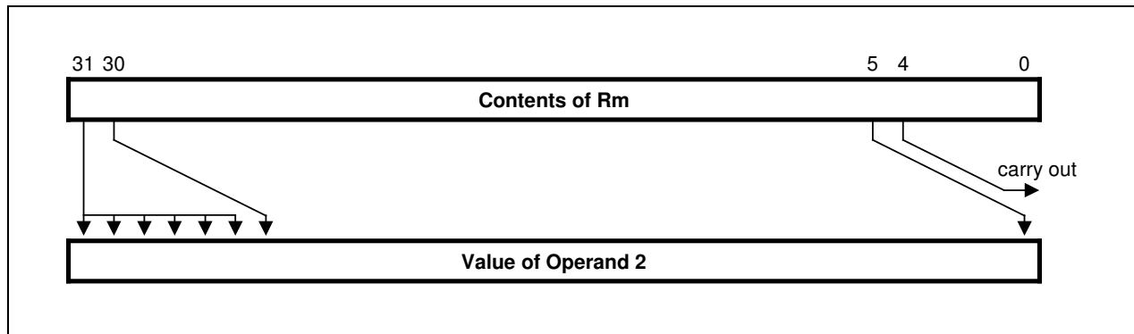
Figure 3-8. Arithmetic Shift Right
