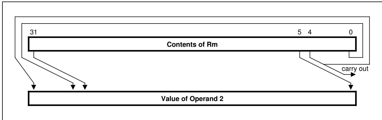
Figure 3-9. Rotate Right
